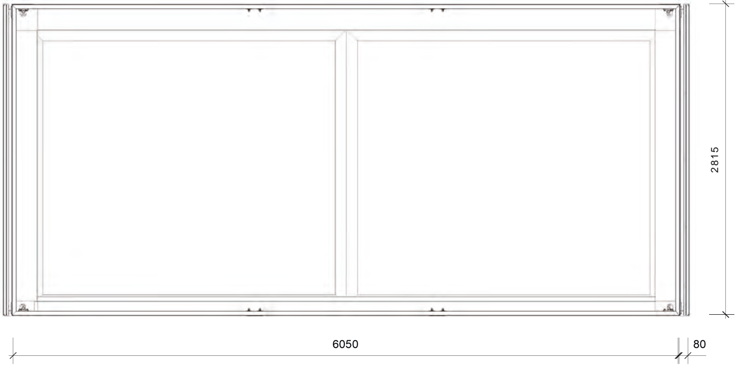
Container Längsseite
