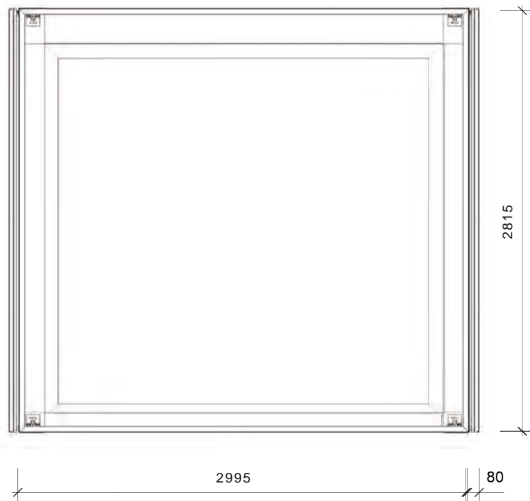
Container Stirnseite
